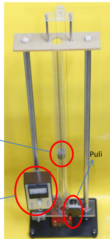
Hình 2. Hệ thí nghiệm
